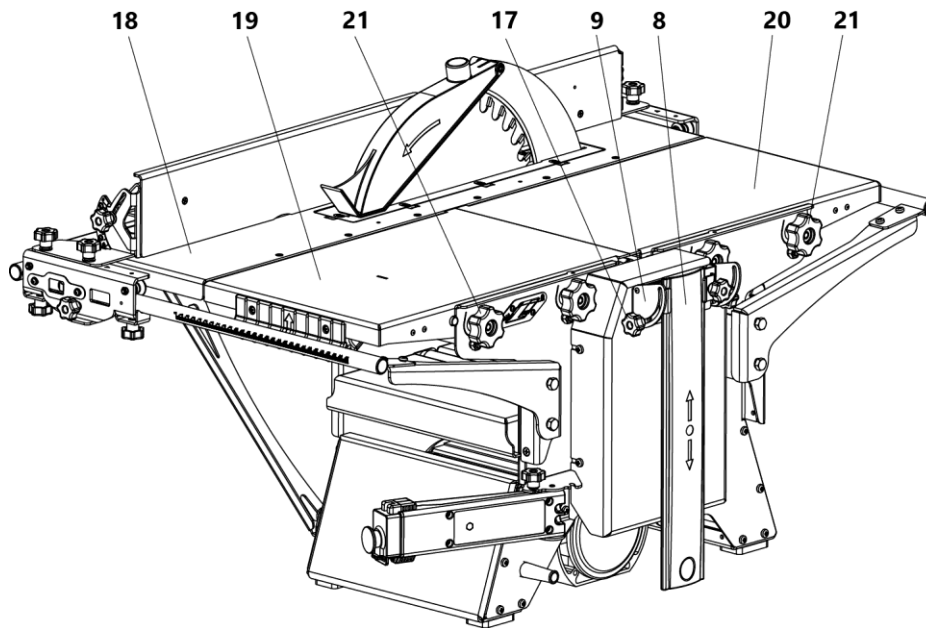
Рис. 11 Станок в режиме пиления с установленной линейкой комбинированной слева от пильного диска 8 – ограждение ножевого вала; 9 – кронштейн; 17 – винт-барашек; 18 – стол пильный; 19 – стол загрузочный; 20 – стол приёмный; 21 – гайка-барашек
