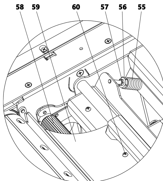
Рис. 28 Регулировка подающего вала 55 – пружина; 56 – гайка; 57 – контргайка; 58 – подающий вал; 59 – защитный кожух подающего вала; 60 – винт
