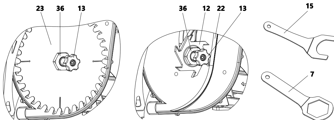
Рис. 14 Демонтаж пильного диска. Установка фрезы 7 – ключ кольцевой; 12 – фреза дисковая; 13 – гайка-барашек регулировки глубины пропила; 15 – ключ рожковый; 22 – вкладыши для фрезерования; 23 – диск пильный; 36 – гайка зажимная
